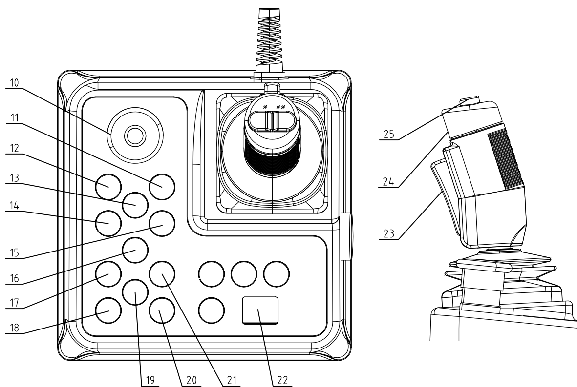
手柄总成
