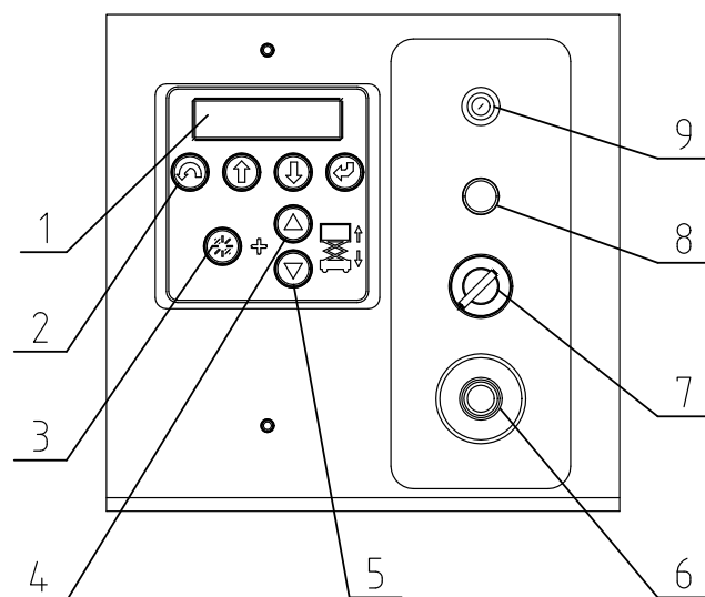
下控制面板
